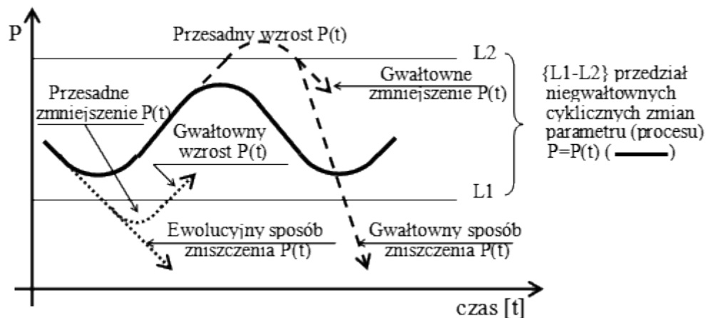
Rys.1. Ilustracja podstawowych relacji pomiędzy cyklicznymi i monotonicznymi procesami
